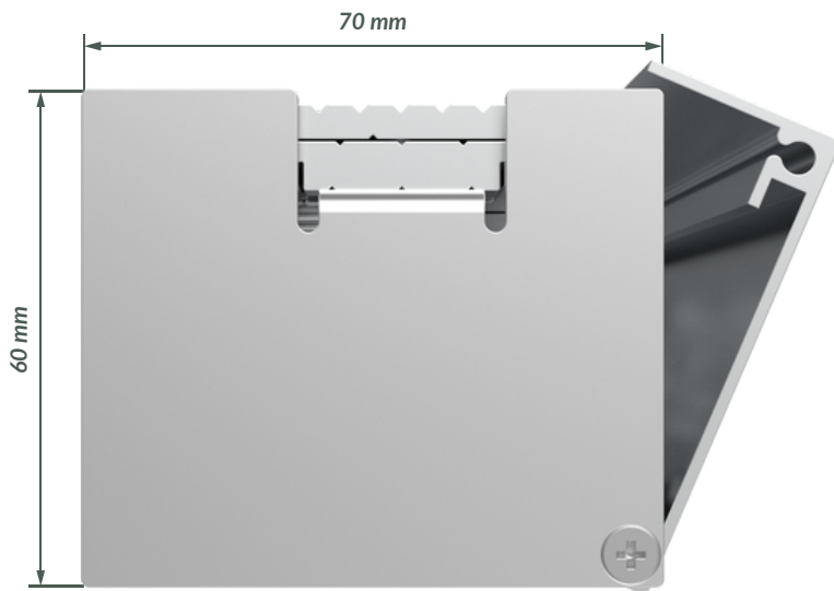
Tényleges méretarány 1:1
